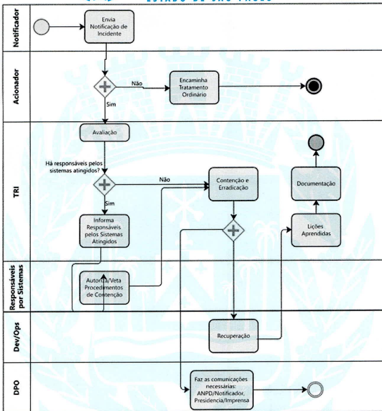
Diagrama BPMN do processo de resposta a Incidentes
